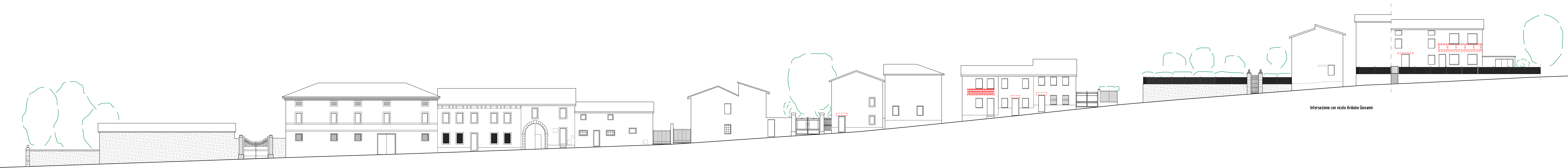
Prospetto di progetto - Via Vescove Carlussare lato sud
